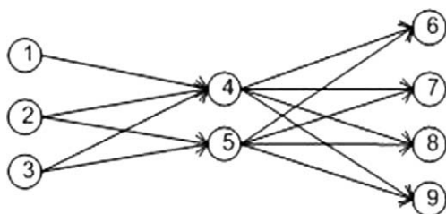
Fig. 1. Graph G.
